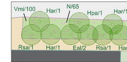
DETAIL ZÁHONU 1, 1:100
